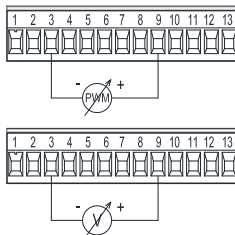
Figura 8: Morsettieria estraibile 13 poli: ingressi 0-10V e PWM
