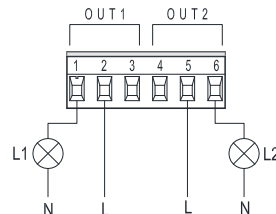
Resim 9: 6 kutuplu çekmeceli klemens kutusu: Çıkışlar bağlantı örneği
