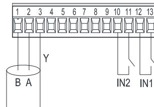
Εικόνα 7: Αφαιρούμενη κλέμμα 13 πόλων: ψηφιακές εισόδους και MODBUS
