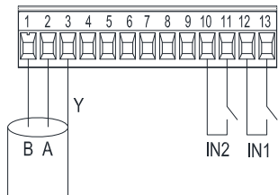
Attēls 7: Iznemams spaiļu panelis ar 13 kontaktiem: digitālās ieejas un MODBUS
