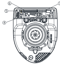
Slika 5: Električni priključki (zadaj)
