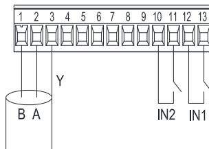
Figura 7: Barra de terminais extraível 13 pínos entradas digitais e MODBUS
