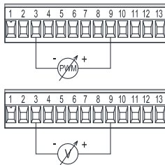
Obr. 8: Vyjímátná 13 pólová svorkovnice: vstupy 0-10V a PWM
