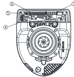
Εικόνα 5: Ηλεκτρική συνδεσμολογία (πίσω μέρος)
