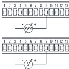
Attēls 8: Izmēams spaiļu panelis ar 13 kontaktiem: ieejas 0-10V un PWM
