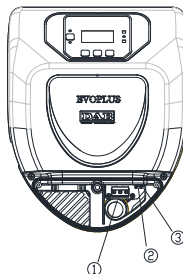
Abbildung 4: Elektroanschlüsse (Frontseite)
