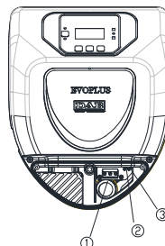
4 pav. Elektros jungtis (priekis)
