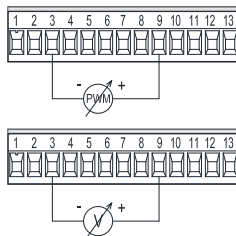
Figur 8: Udtagelig 13-polet klemliste: 0-10V indgange og PWM
