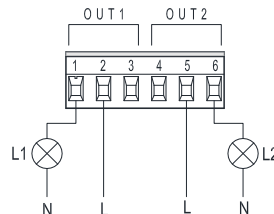
Kuv. 9: 6-napainen ulosvedettävä riviliitin: esimerkki lähtöjen kytkennästä
