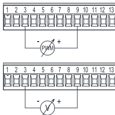
Εικόνα 8: Αφαιρούμενη κλέμμα 13 πόλων: είσοδο 0-10V και PWM
