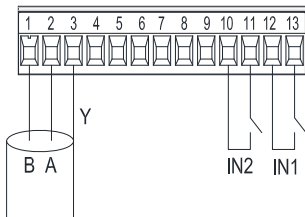
Figura 7: Cutie cu bome extractibile 13 poli intrări digitale și MODBUS
