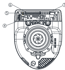
Figura 5: Conexiuni electrice (spate)
