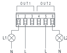
Сх. 9: Знімна клемна колодка 6 полюсів: приклад приєднання виходів
