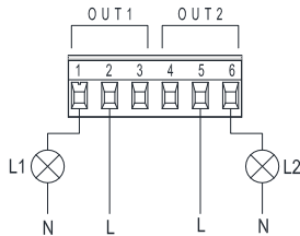
Attēls 9: Izmēams spaiļu panelis ar 6 kontaktiem: izeju savienošanas piemērs
