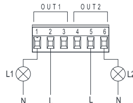
Obr. 9: Vyberateľná 6-pólová svorkovnica: príklad zapojenia výstupov
