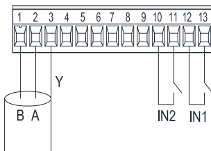
Figur 7: Udtagelig 13-polet klemmiste: digitale indgange og MODBUS
